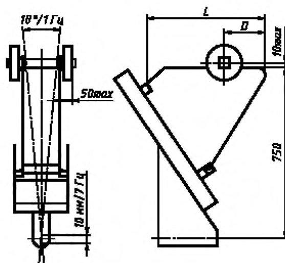
Рисунок 3 — Динамические испытания
