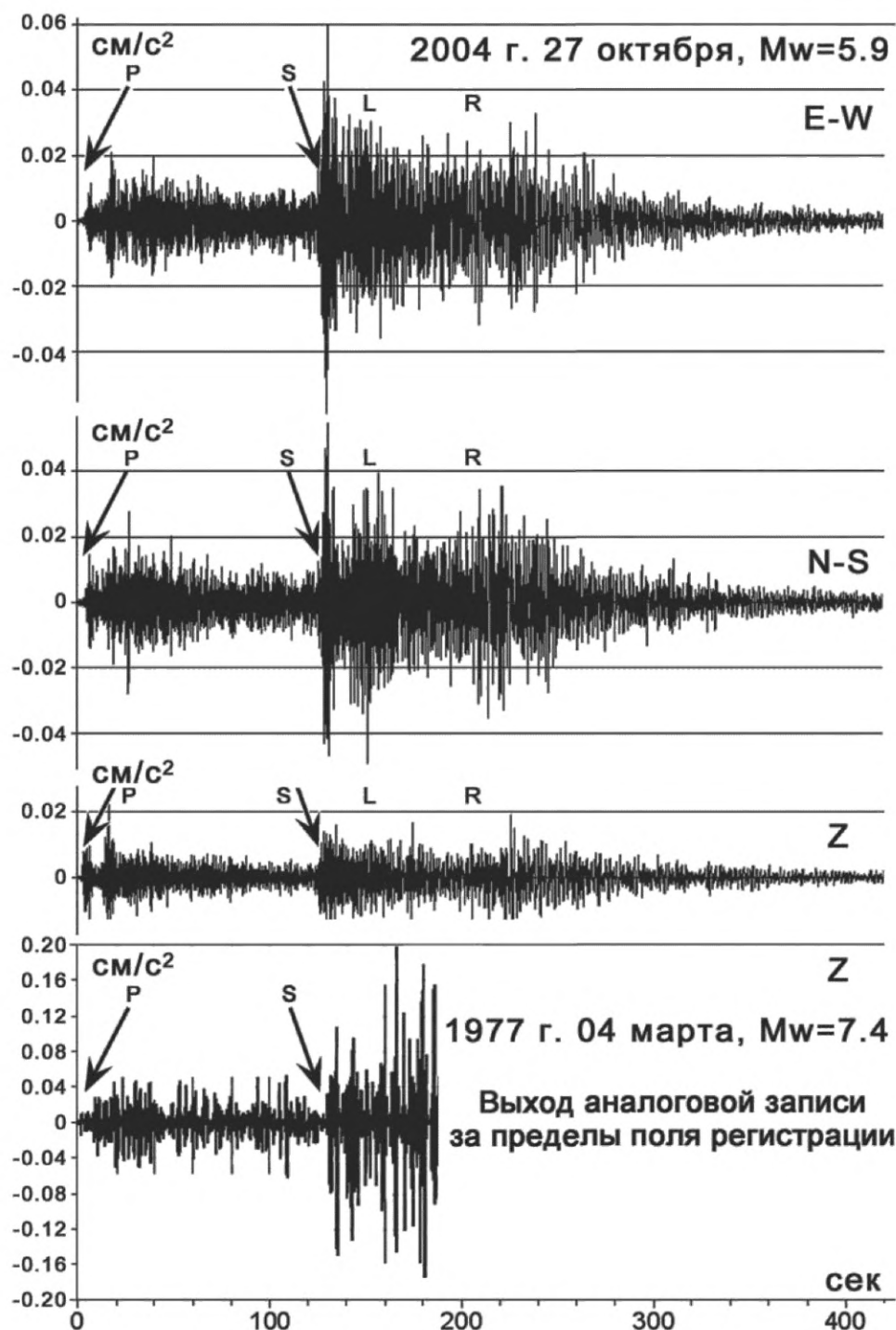
Рисунок 5 — Цифровая трехкомпонентная акселерограмма движений грунта под сейсмостанцией «Москва» во время Вранчского землетрясения 27 октября 2004 г. (магнитуда M_w = 5,9 ) и фрагмент вертикальной составляющей акселерограммы при самом сильном за последние 60 лет Вранчском землетрясении 4 марта 1977 г. с M_w = 7,4 (внизу). Указано время прихода на центральную сейсмическую станцию «Москва» продольных (P), поперечных (S) и поверхностных сейсмических волн Лява (L) и Релея (R). Сейсмометрическая аппаратура станции расположена в подвальном помещении на глубине 4 м от земной поверхности, где: E-W — восток — запад; N-S — север — юг; Z — вертикальная составляющая
