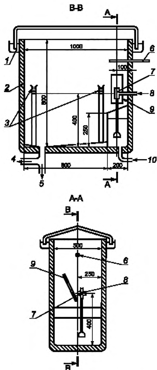
1 -- гидроаккумулятор; 2 -- нагревающая теплоизоляционная стенка; 3 -- сборники (воронка площадью 80 см 2 ); 4 -- отвод воздуха; 5 -- отвод воды; 6 -- термометр; 7 -- отверстие распылителя (сопло); 8 -- подвод сжатого воздуха; 9 -- дефлектор с регулируемым наклоном и расстоянием; 10 -- подвод соляного раствора
