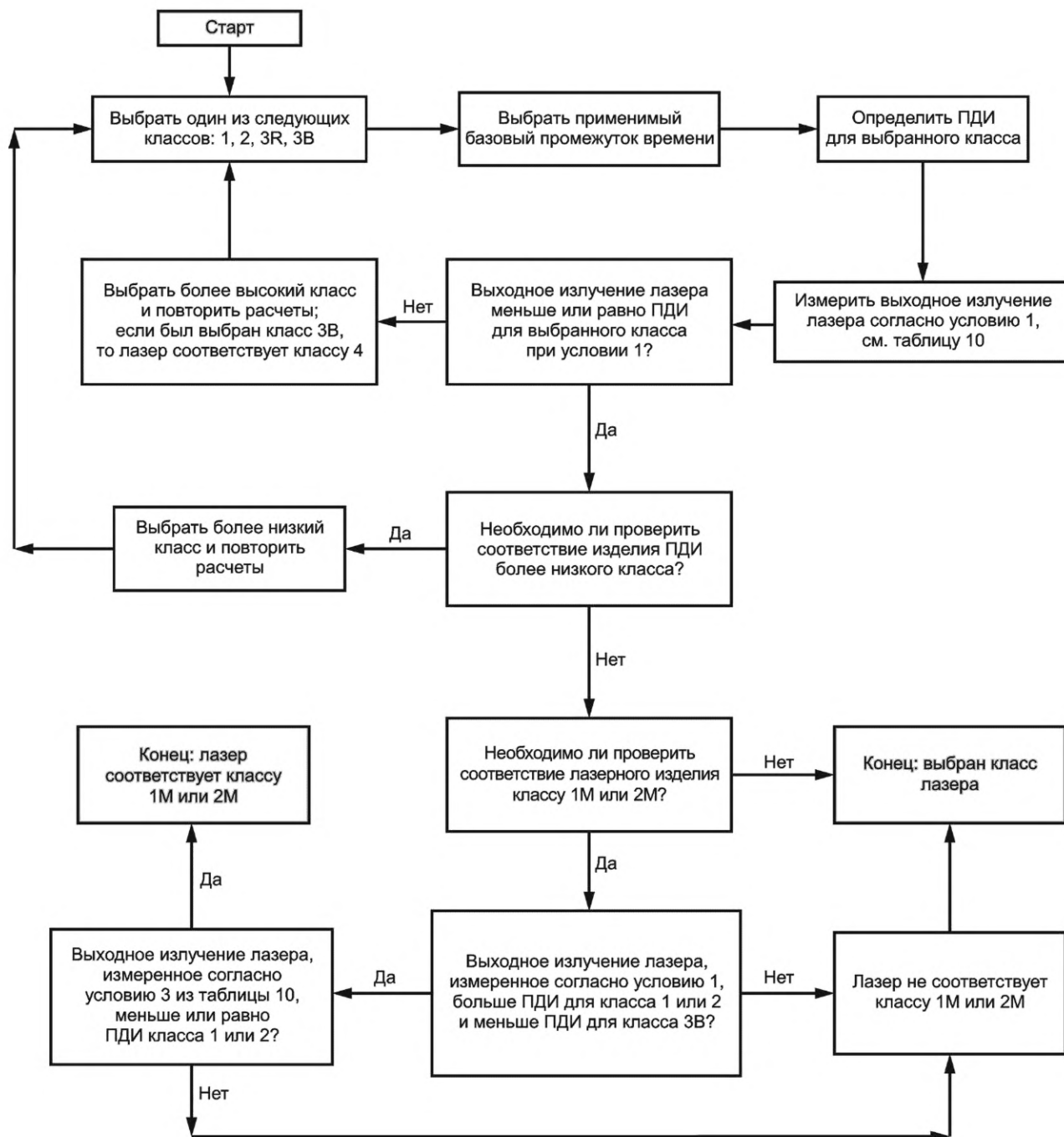
Рисунок В.2 — Инструкция в виде блок-схемы по классификации лазерных изделий классов 1М и 2М
