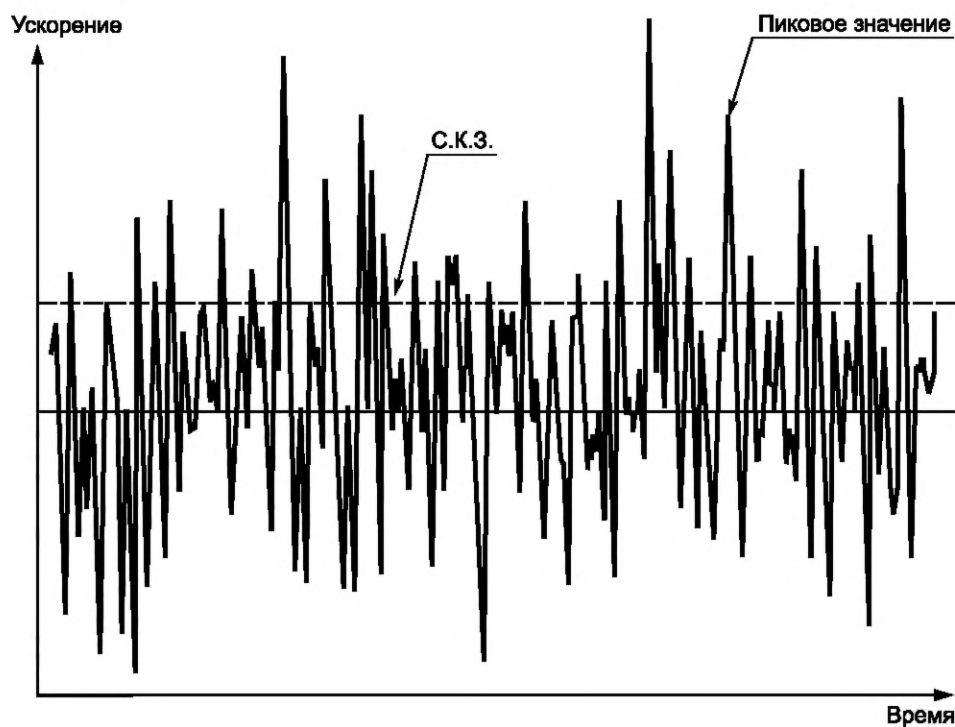
Рисунок 2 — Отсечка (ограничение) сигнала
