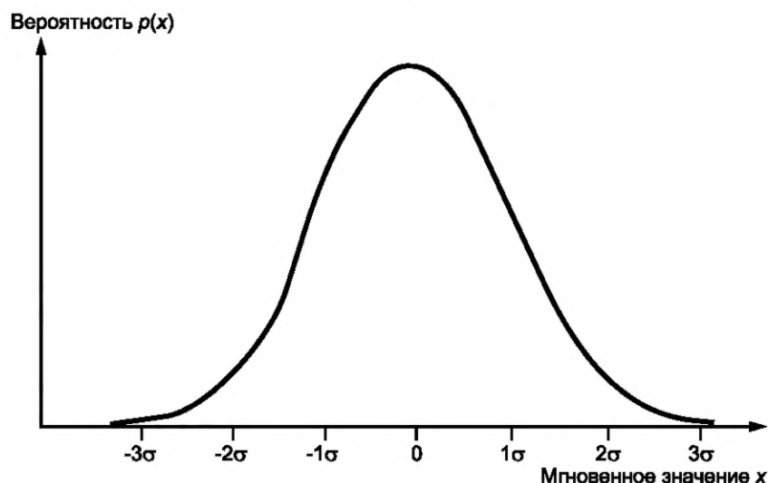
Рисунок 1 — Гауссовская плотность распределения вероятностей
