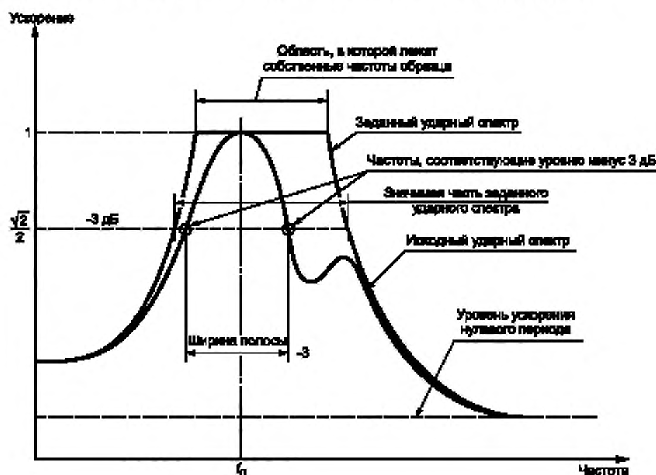
Рисунок 3 — Типичная огибающая спектра ответа
