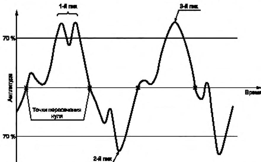
Рисунок 2 — Пример обнаружения пиков отклика, превышающих пороговое значение (70 %)
