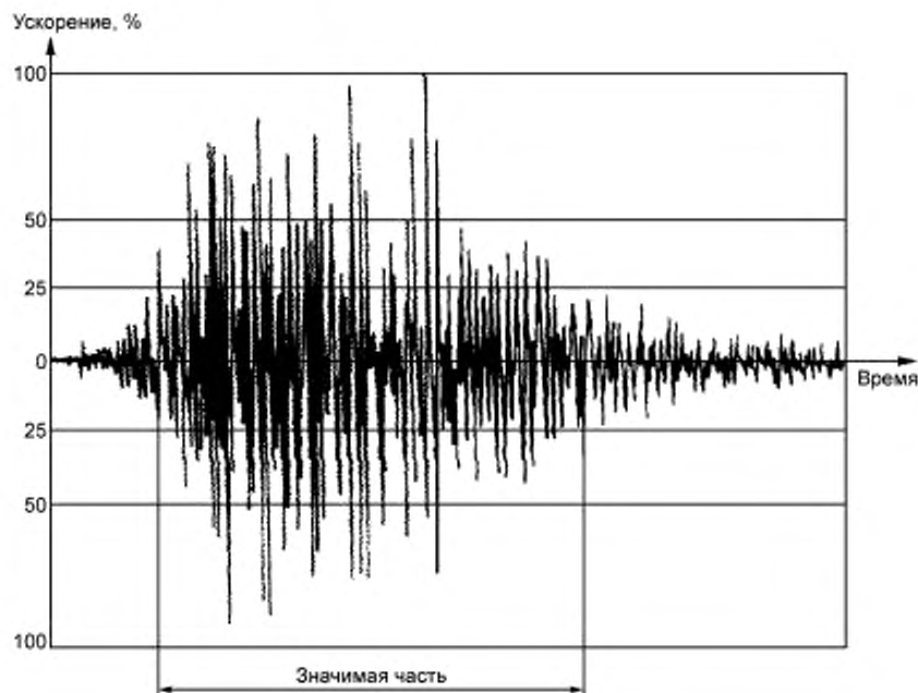
Рисунок 4 — Типичная форма акселерограммы
