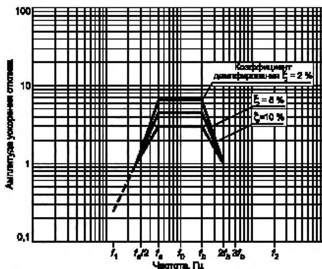
Рисунок — Категория 2. Рекомендуемый вид заданного спектра ответа
