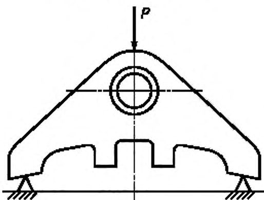
Схема ударных испытаний
