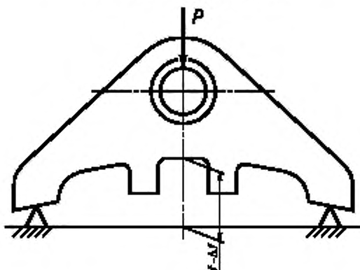
Схема испытания на жесткость
