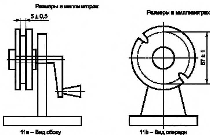
Рисунок 11 — Устройство для намотки
