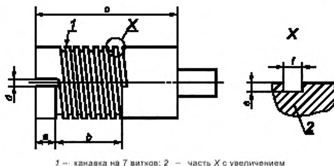
Рисунок 2 — Конструкция и размеры оправки
