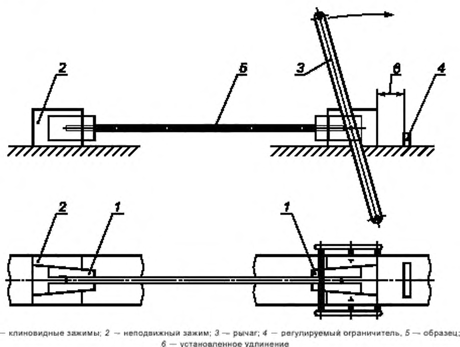
Рисунок 5 — Устройство для испытания рывком
