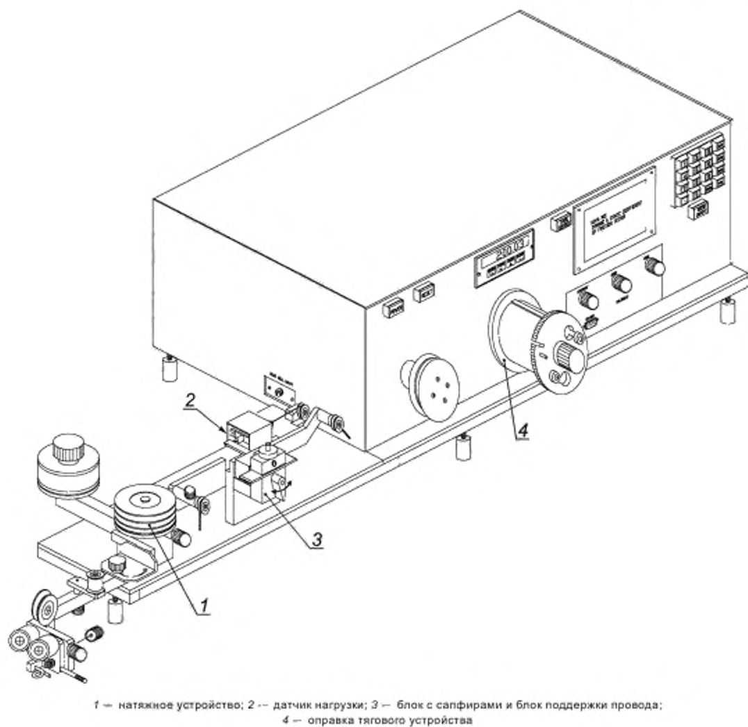
Рисунок В.3 — Типовое испытательное устройство для определения динамического коэффициента трения
