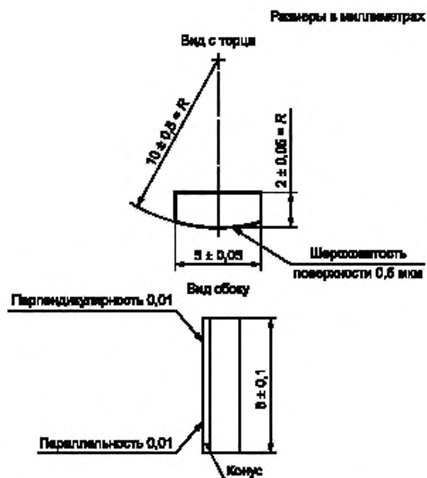
Рисунок В.4 — Материал — сапфир (синтетический)
