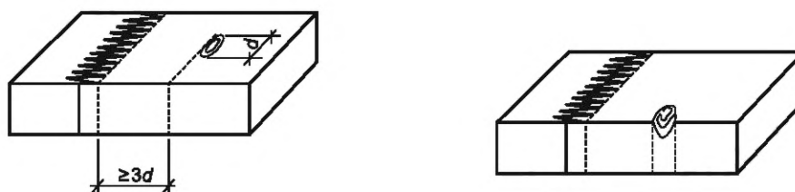
Рисунок 3 — Минимальное расстояние от сучка до основания зубчатого шипа
