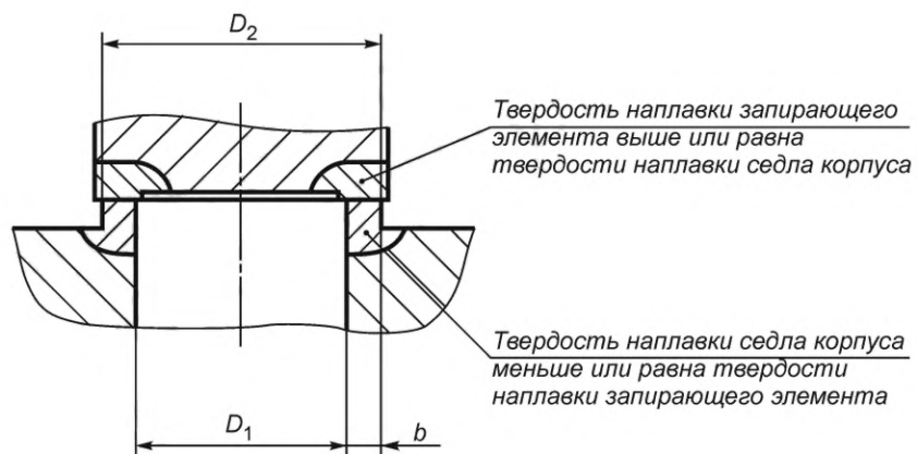
Рисунок Е.1 — Плоское уплотнение в затворе
