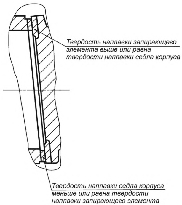
Рисунок Е.4 — Уплотнение в затворе клиновых задвижек
