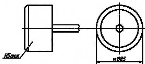
Рисунок 3 — Размеры молотка
