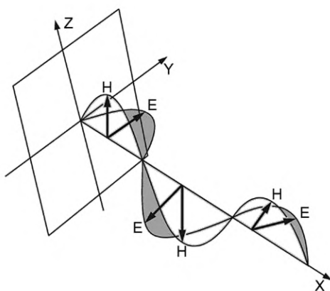
Рисунок 2 — Электромагнитное поле
