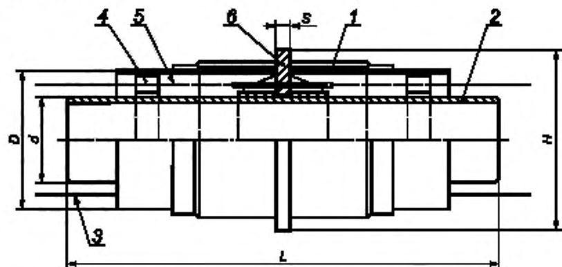
1 — ПЭ-оболочка; 2 — стальная труба; 3 — проводник—индикатор СОДК; 4 — центрирующая опора; 5 — изоляция из ППУ; 6 — неподвижная опора
