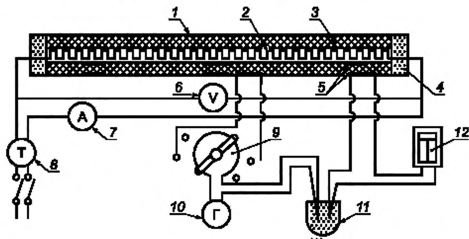
1 — стальная труба; 2 — электронагреватель; 3 — испытуемый материал; 4 — охранный секция; 5 — термодатчики; 6 — вольтметр; 7 — амперметр; 8 — автоматический выключатель; 9 — переключатель; 10 — гальванометр; 11 — сосуд со льдом; 12 — самопишущий гальванометр
