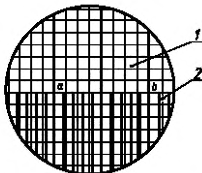
1 — сетка окулярного микрометра; 2 — шкала объекта-микрометра
