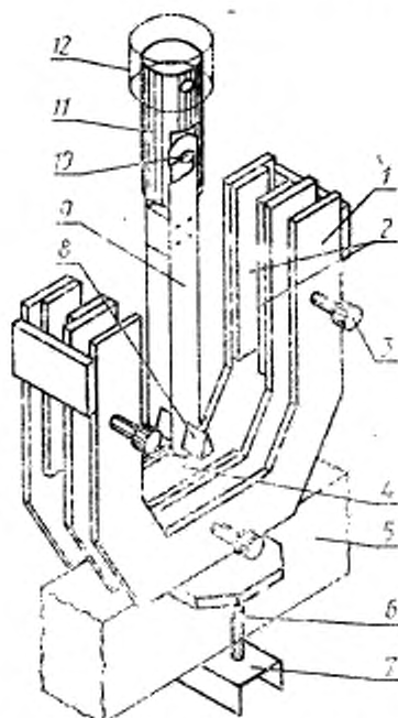
1 — корпус зажимов; 2 — продольные зажимы; 3 — прижимные винты; 4 — поперечный зажим; 5 — подающая траверса разрывной машины; 6 — шпилька; 7 — планка; 8 — раздирающий стержень; 9 — скоба; 10 — штифт; 11 — стержень; 12 — соединительный узел разрывной машины
