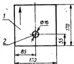
1 — элементарная проба; 2 — отверстие
