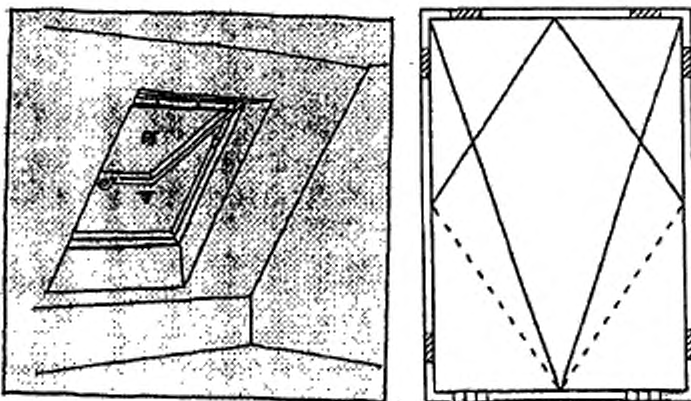
б — с комбинированным открыванием
