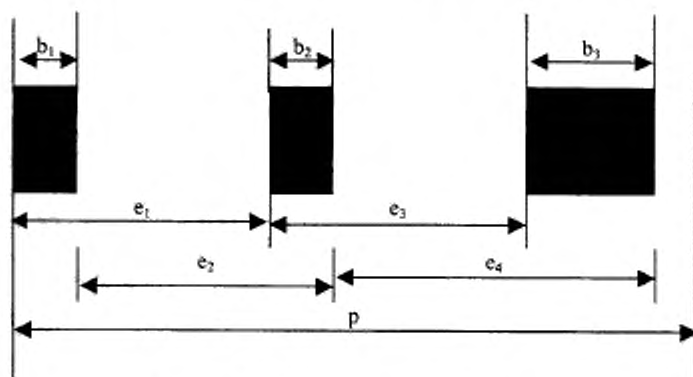
Рисунок 5 — Декодирование размеров
