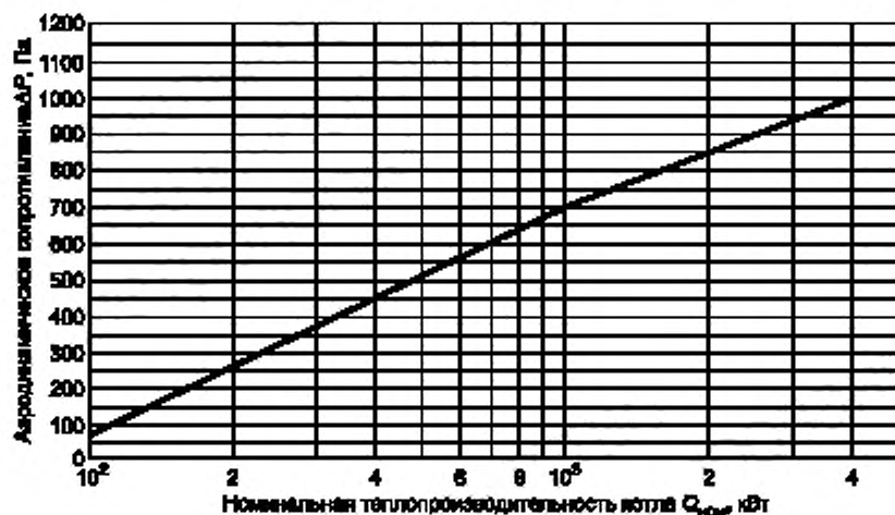
Рисунок 3 — Максимальное аэродинамическое сопротивление котла на принудительной тяге или под наддувом
