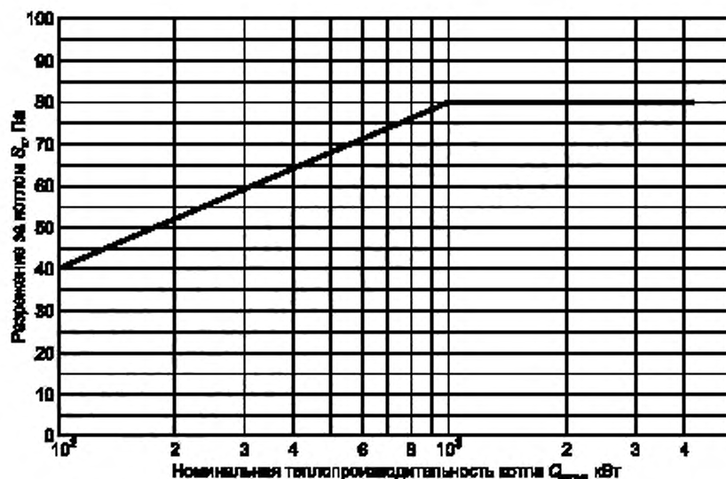
Рисунок 2 — Максимальное разрежение за котлом на естественной тяге
