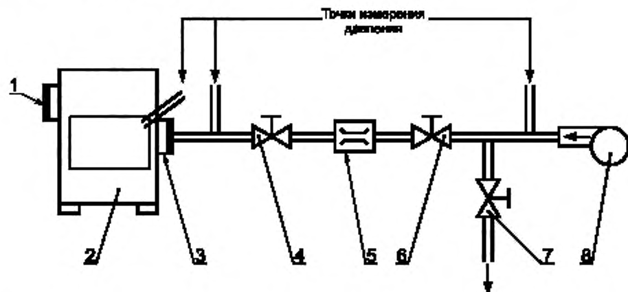
1 — патрубок входящих газов; 2 — испытываемый котел; 3 — амбразура горелки; 4 — регулирующий орган 1; 5 — измеритель расхода; 6 — регулирующий орган 2; 7 — регулирующий орган 3; 8 — вентилятор
