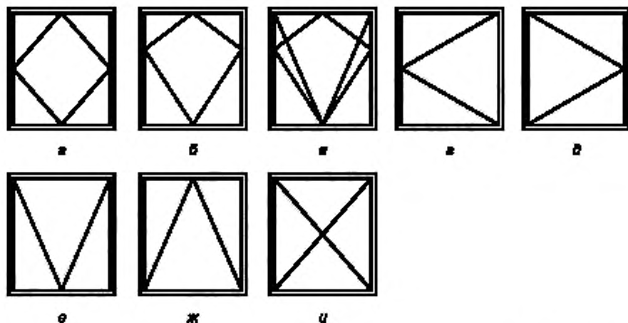
а — среднесповоротное открывание створки по центральной оси; б — среднесповоротное открывание створки со смещенной осью; в — комбинированное открывание; г, д — распашное боковое открывание; е — верхнеподвесное открывание; ж — откидное открывание по нижней оси; и — неоткрывающаяся створка (глухое)
