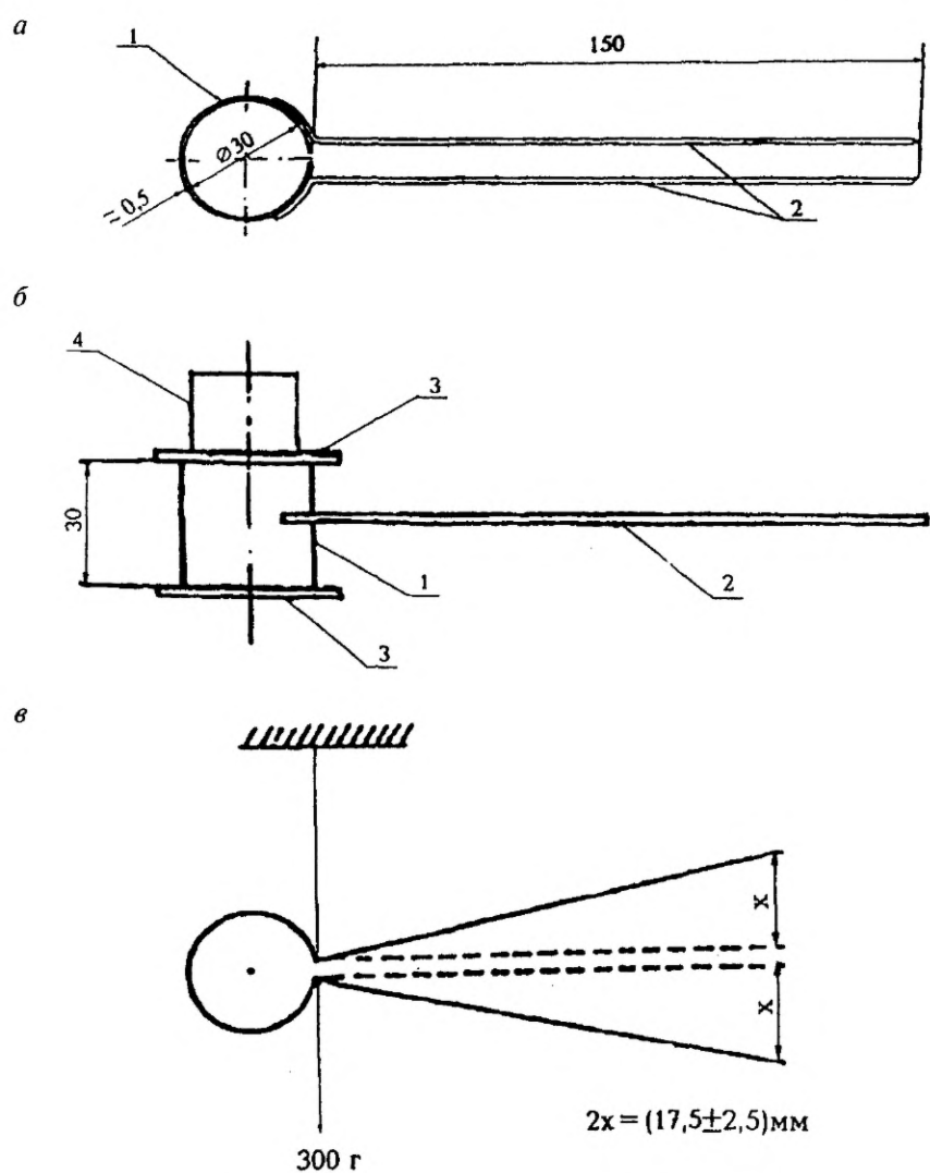
а — кольцо Ле Шателье (вид сверху); б — кольцо Ле Шателье с пластинками и пригрузом (вид сбоку); в — схема проверки упругости кольца Ле Шателье 1 — кольцо с прорезью; 2 — индикаторная игла; 3 — пластинка; 4 — пригруз»
