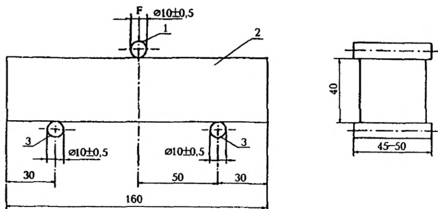
Рисунок 10 — Схема расположения образца-балочки при испытании на изгиб
