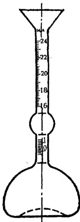
Рисунок 1 — Прибор Ле Шателье
