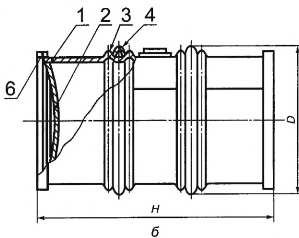
1 — корпус; 2, 5 — донья; 3 — зиг; 4 — обруч катания; 6 — обруч концевой а — бочка со сливоналивной горловиной на верхнем дне; б — бочка со сливоналивной горловиной на корпусе
