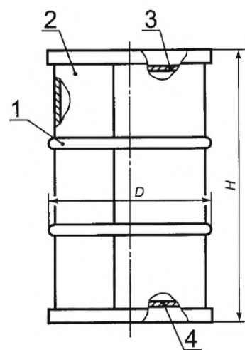
1 — гофр; 2 — корпус; 3, 4 — донья
