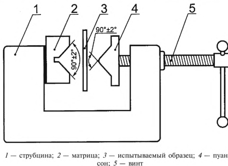
Рисунок 13 — Устройство для загиба образца (пластины)
