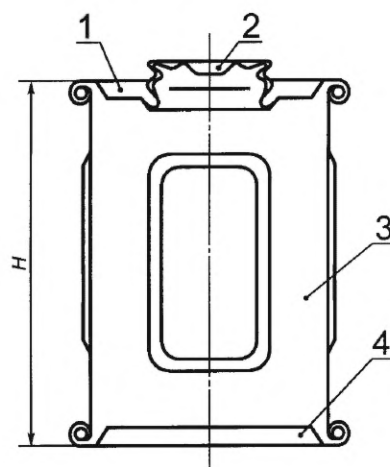
Рисунок 6 — Фляга типа II с опорными обручами
