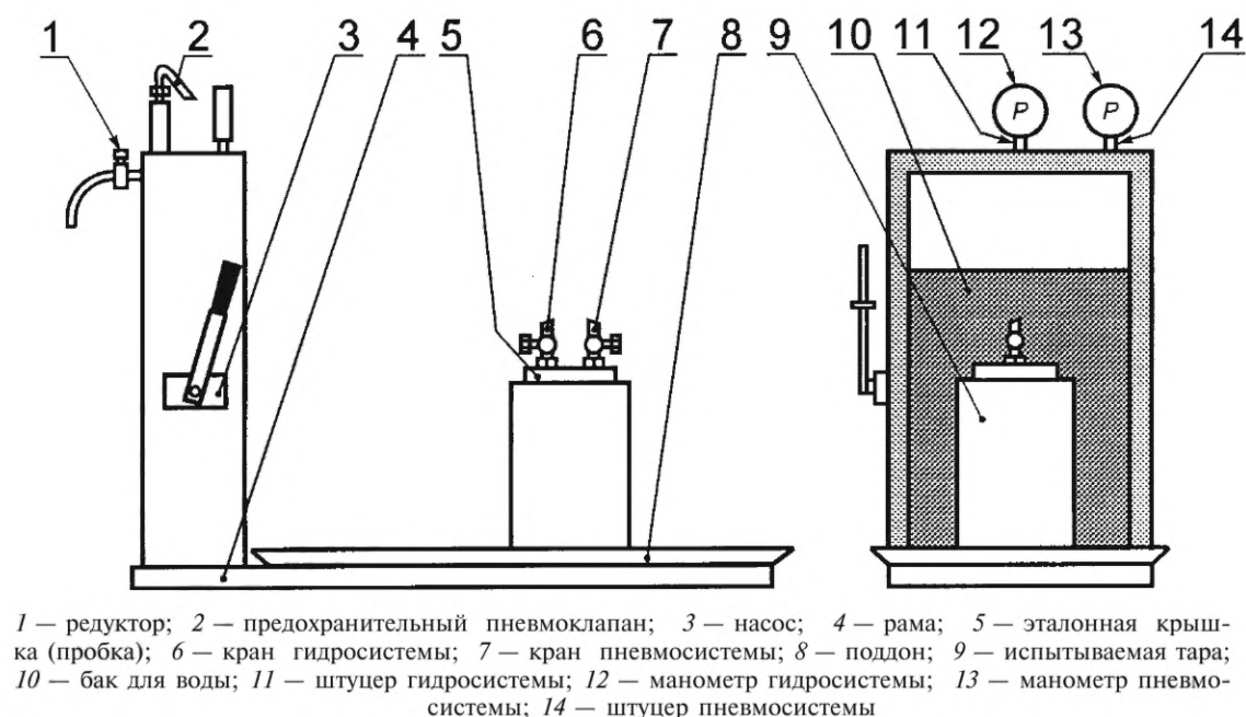
Рисунок 11 — Схема стенда для испытания тары на герметичность и гидравлическое давление
