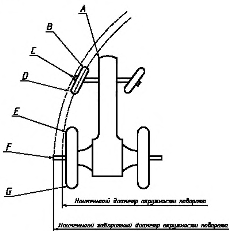
Рисунок 1 — Схема определения диаметров окружности поворота
