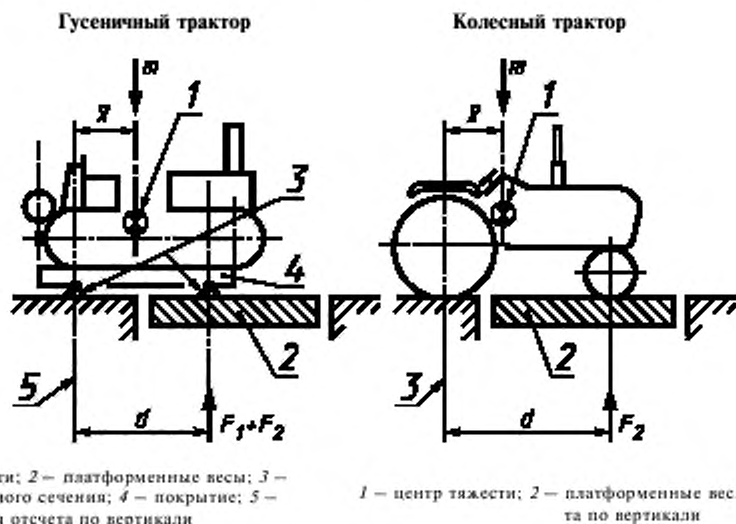
Рисунок 1 — Определение горизонтальной продольной координаты x
