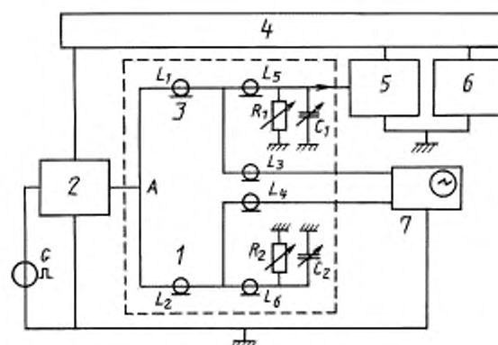
1, 3 — согласованное T-образное соединение; 2 — цепь управления на входе; 4 — источник питания; 5 — измеряемая схема; 6 — дополнительная цепь нагрузки; 7 — осциллограф
