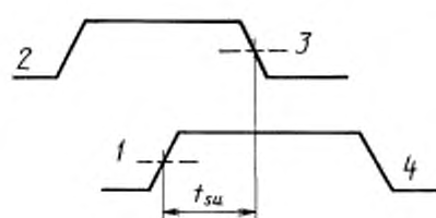
Время установления (типичные формы сигнала)
