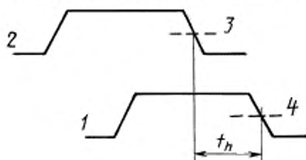
Время удержания (типичные формы сигнала)
