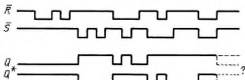
Временная диаграмма
