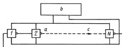
Кольцевой генератор для инвертирующих N-схем
