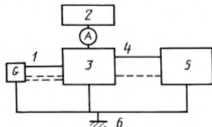
G — источник напряжения и генератор импульсов; 1 — вход(ы); 2 — источник питания; 3 — измеряемая схема; 4 — выход(ы); 5 — цепь на выходе; 6 — опорная шина
