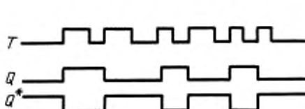
Временная диаграмма
