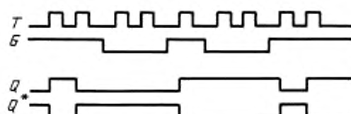
Временная диаграмма
