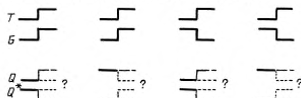
Функциональные (последовательностные) матрицы T_G -схемы с задержкой по входу T по отношению ко входу G
