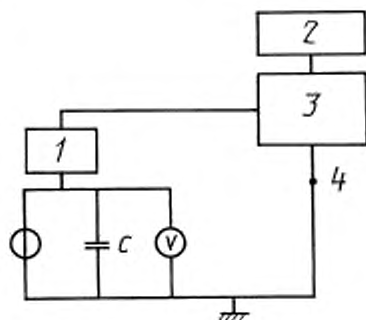
1 — высокочастотный мост; 2 — источник питания; 3 — измеряемая интегральная схема; 4 — контрольная точка
