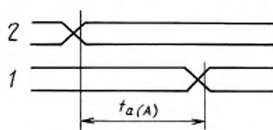
Измерение времени выборки адреса
