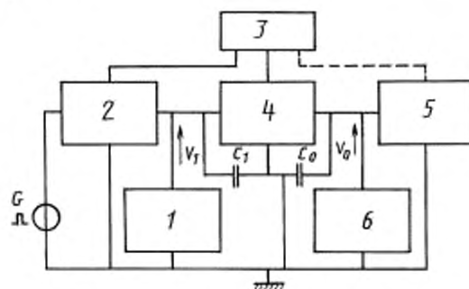
1 — прибор для измерения времени; 2 — цепь управления; 3 — источник питания; 4 — измеряемая интегральная схема; 5 — цепь нагрузки; 6 — прибор для измерения напряжения
