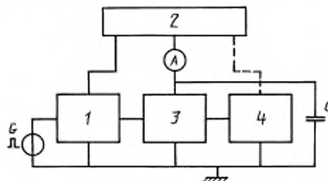
1 — цепь(и) управления на входе; 2 — источник питания; 3 — измеряемая схема; 4 — цепь(и) нагрузки на выходе
