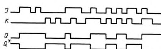
Временная диаграмма
