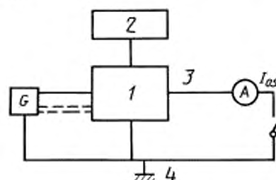
G — источник напряжения и генератор импульсов; 1 — измеряемая схема; 2 — источник питания; 3 — измеряемый выход; 4 — опорная шина
