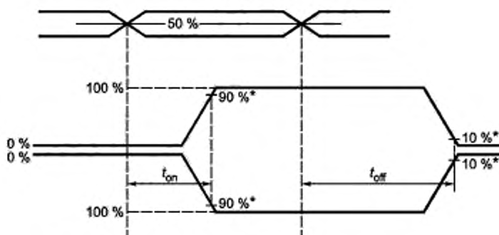
Измерение времени включения и выключения схем переключения аналоговых сигналов
