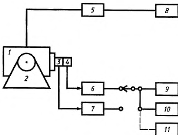
1 — вибростенд; 2 — опора вибростенда; 3 — эталонный датчик; 4 — калируемый датчик; 5 — усилитель мощности; 6 — согласующий усилитель калируемого датчика; 7 — согласующий усилитель эталонного датчика; 8 — низкочастотный генератор сигналов; 9 — электронный вольтметр; 10 — измеритель нелинейных искажений; 11 — электронный осциллограф
