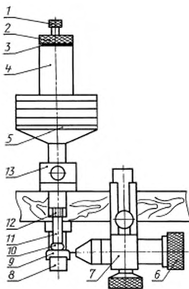
1 — клапан; 2 — пробка; 3 — прокладка; 4 — корпус; 5 — съемные грузы; 6 — держатель; 7 — струбцина; 8 — плата с желобом; 9 — изделие; 10 — ватный тампон; 11 — хлорвиниловая трубка; 12 — ниппель; 13 — направляющая ручка
