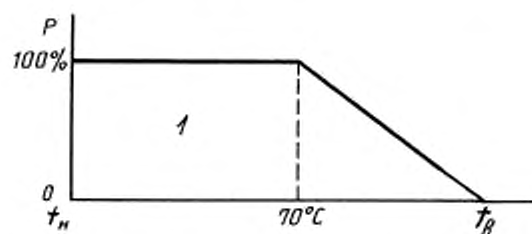
1 — рекомендуемая зона эксплуатации; t_n — нижняя температура категории; t_v — верхняя температура категории
