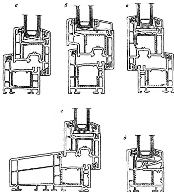
а — оконная система из трехкамерных профилей; б — оконная система с четырехкамерной створкой и трехкамерной коробкой (расположение наружных стенок створки и коробки в одной плоскости); в — оконная система из трехкамерных профилей (открывание наружу); г — оконная система из многокамерных профилей с расширенной коробкой; д — оконная система с остекленной коробкой
