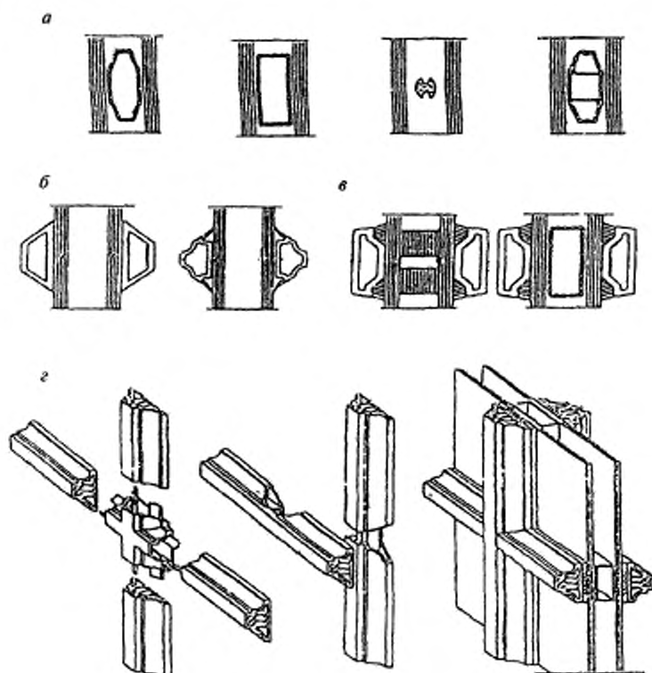
a — профили внутренней рамки стеклопакета; б — накладные декоративные раскладки; в — вариант комбинированного применения накладных раскладок и внутренней рамки стеклопакета; з — переплетные соединения раскладок
