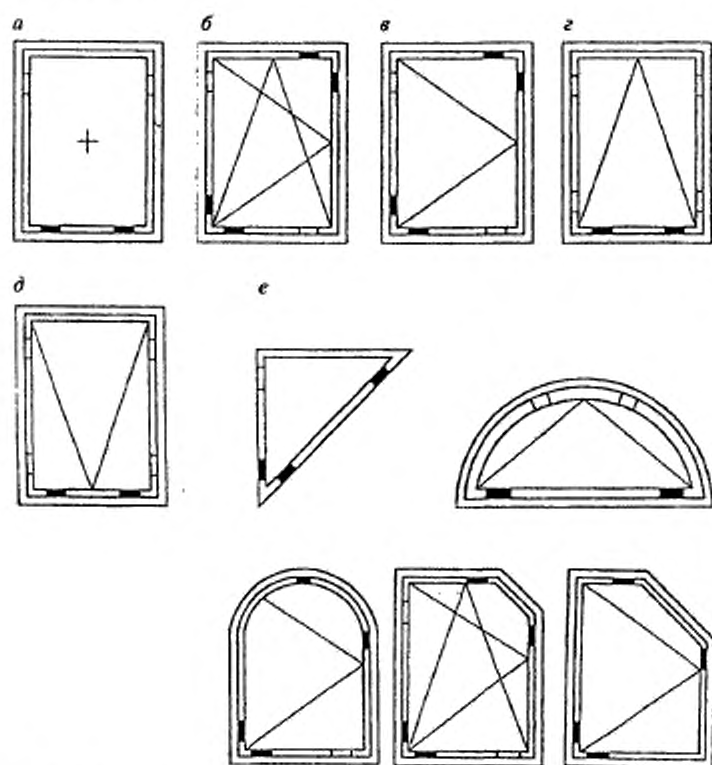
Виды открывания оконных блоков: а — неоткрывающиеся; б — поворотно-откидное; в — поворотно-откидное (распашное); г — откидное; д — подвесное; е — установка подкладок в фигурных оконных блоках
