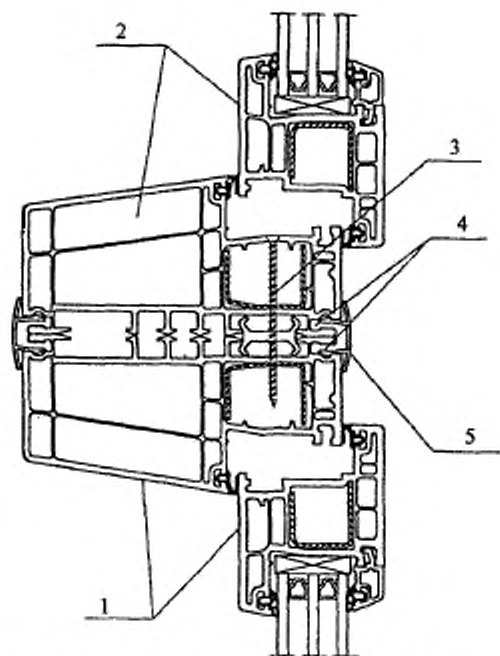
1 — оконный блок; 2 — дверной балконный блок; 3 — стяжной шуруп; 4 — силиконовый герметик; 5 — нащельник
