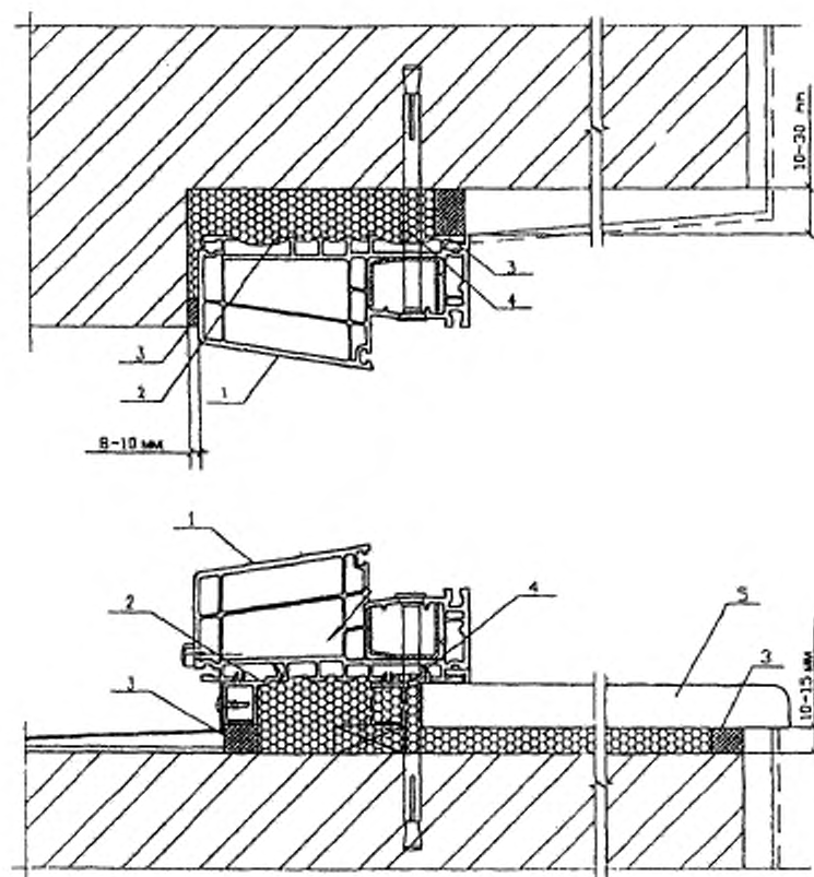
1 — оконная коробка; 2 — пеноутеплитель; 3 — уплотняющая прокладка; 4 — монтажный дюбель; 5 — подоконная доска
