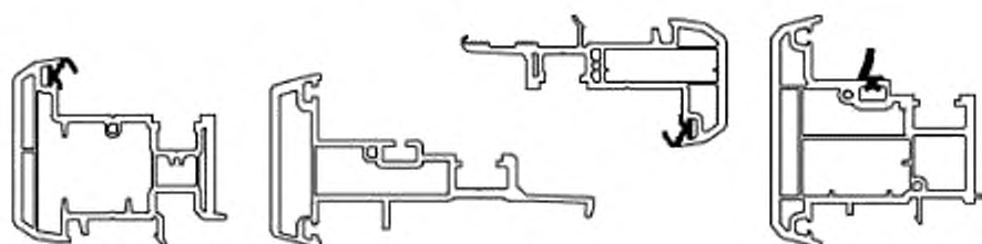
Сечения профилей штаплов
