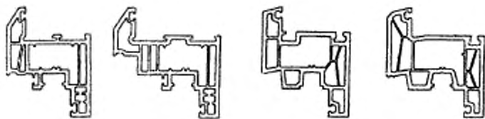
Сечения профилей створок
