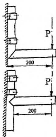
Рисунок 4 — Определение прочности угловых сварных соединений (для углового соединения под 90^\circ и Т-образного соединения)
