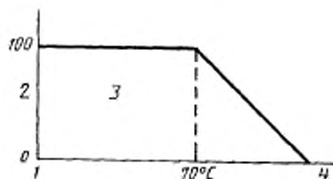
1 — нижняя температура категории; 2 — процент от номинальной мощности рассеяния; 3 — верхняя температура категории; 4 — рекомендуемая зона эксплуатации
