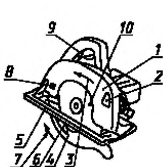
Рисунок 102 — Дисковая пила с внутренним качающимся защитным кожухом
