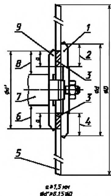
Рисунок 111 — Характеристика фланцев
