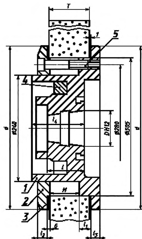
1 — неподвижный фланец; 2 — подвижный фланец; 3 — прокладка; 4 — сегмент; 5 — винт М16-6g × 56.029 по ГОСТ 11738
