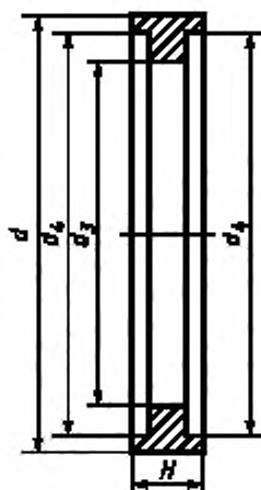
Рисунок 7 — Проставное кольцо
