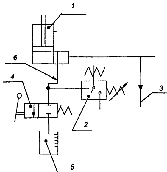
1– гидроцилиндр подъема стрелы; 2 – диагностическое устройство (манометр); 3 – гидрораспределитель; 4 – устройство, имитирующее отказ; 5 – мерный сосуд; 6 – гидролиния связи.
