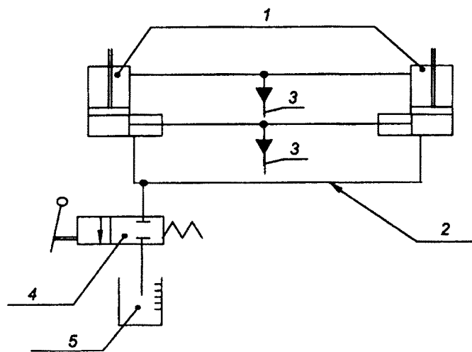
1 – гидроцилиндры подъема стрелы; 2 – гидролиния выравнивания давления; 3 – гидрораспределитель; 4 – устройство, имитирующее отказ; 5 – мерный сосуд;
