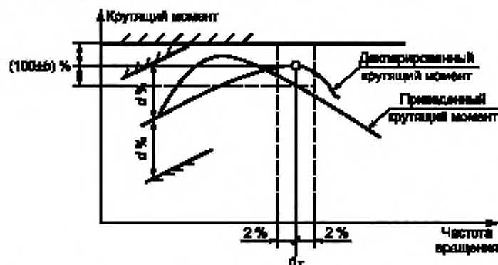
Рисунок 4 — График для декларируемого значения частоты вращения, при которой крутящий момент максимальный
