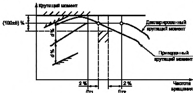
Рисунок 5 — График для декларируемого диапазона частот вращения, при которых крутящий момент максимальный
