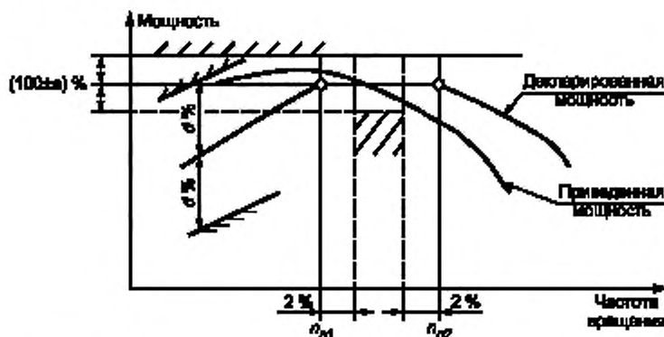
Рисунок 3 — График для декларируемого диапазона частот вращения, при которых мощность максимальная
