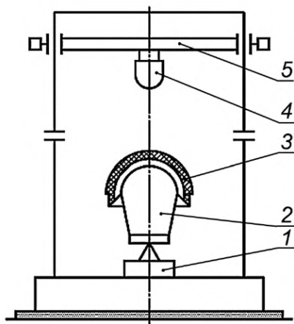
1 — силонизмерительный датчик; 2 — макет головы; 3 — каска; 4 — ударник; 5 — каретка
