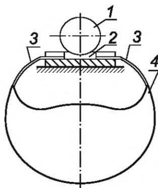
1 — шар; 2 — зажимное замковое устройство; 3 — нижнее ремненное крепление; 4 — каска
