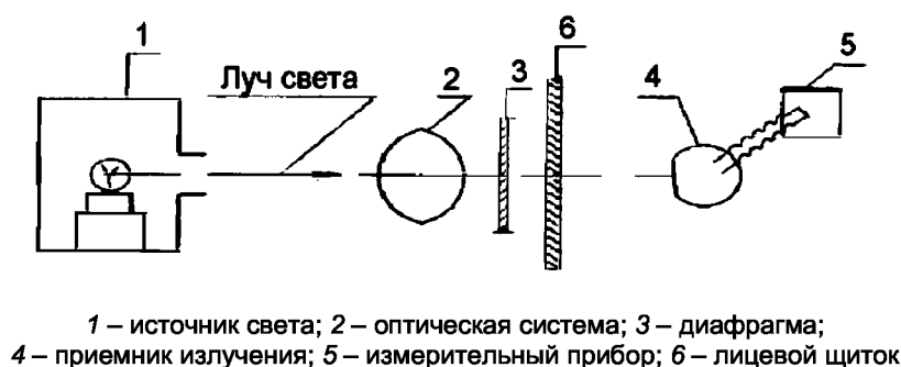
Рисунок 20 – Принципиальная схема стенда
