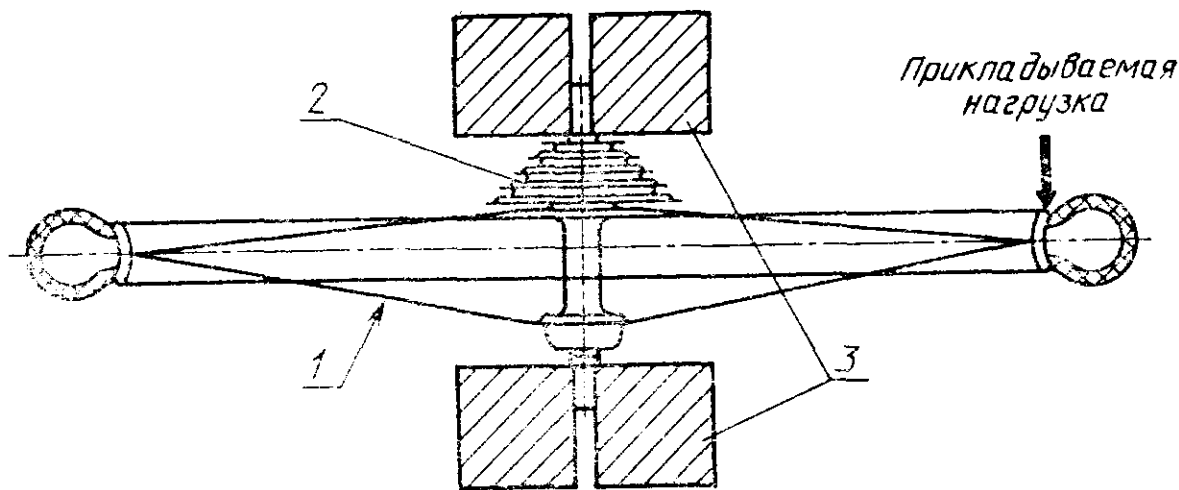
Испытание статической нагрузкой колеса
