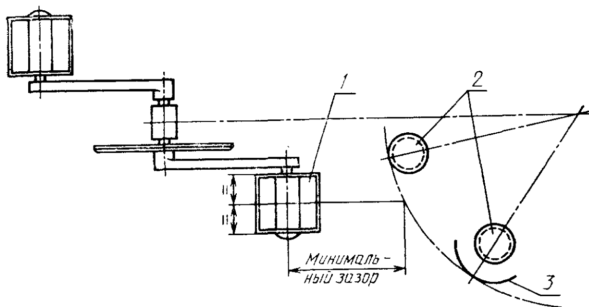
Зазор между педалью и шиной
