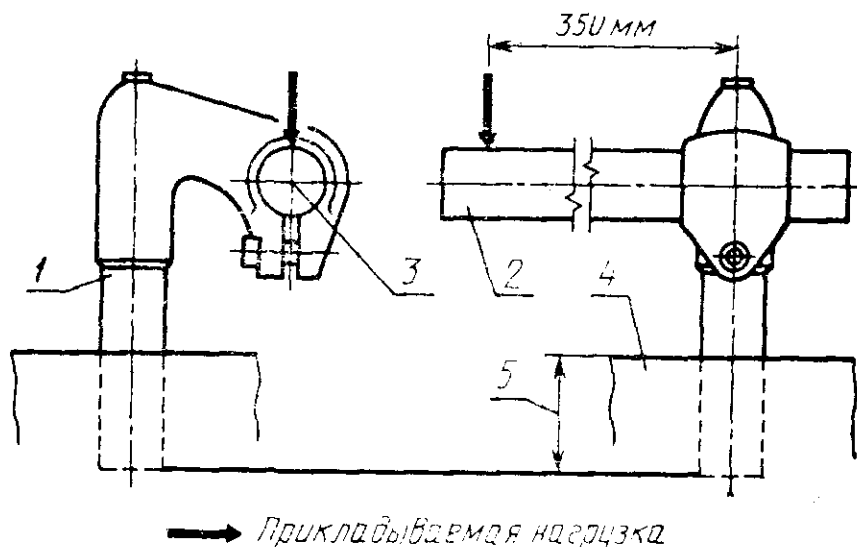
Испытание на кручение стержня руля
