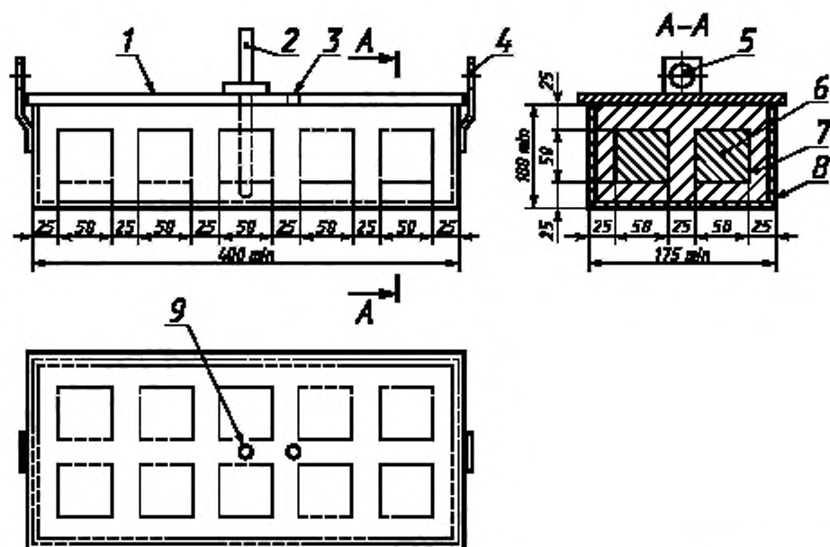
1 — крышка; 2 — термopapa в чехле; 3 — вентиляционное отверстие; 4 — скоба; 5 — отверстие для подъемного стержня; 6 — испытуемый образец; 7 — коксовая засыпка; 8 — камера; 9 — отверстие для термopapa
