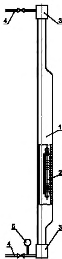
1 — скважинная камера; 2 — пробка; 3 — переходник со штуцерами; 4 — трубопроводы с запорной арматурой; 5 — манометр
