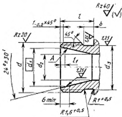
Конструкция и размеры присоединительной части штуцеров клапанов типа 7
