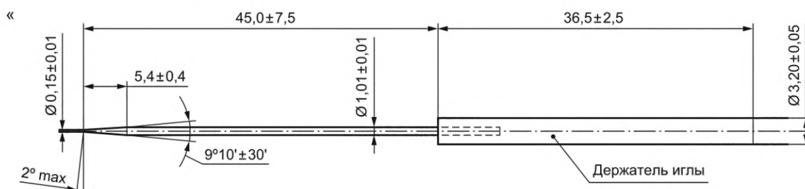
Рисунок 1 — Пенетрационная игла»;
