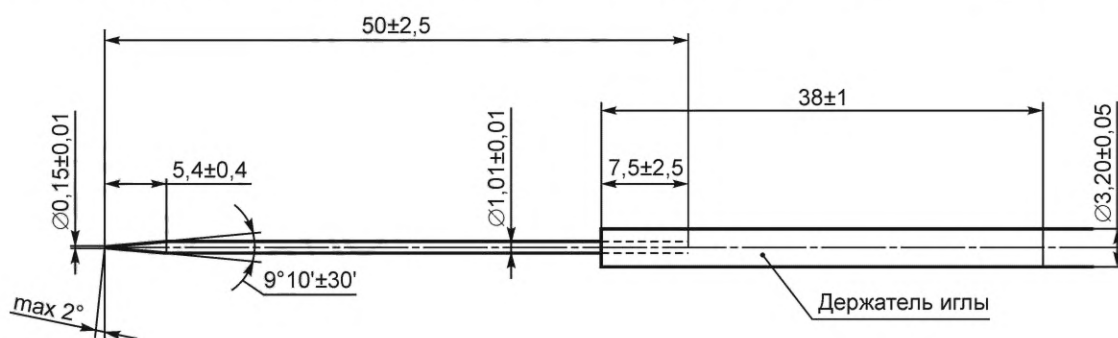
Рисунок 1 — Пенетрационная игла
