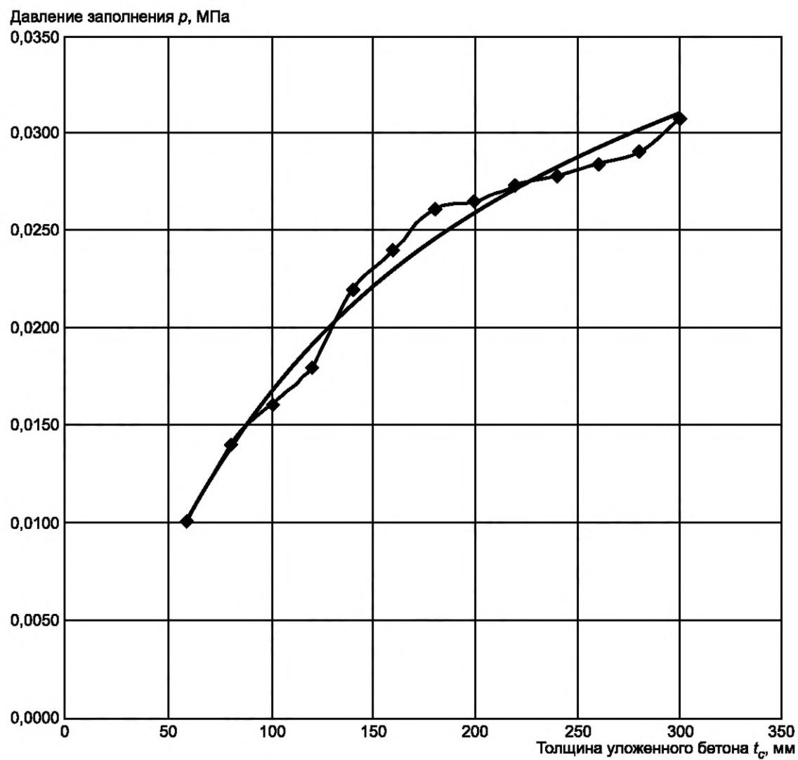
Рисунок Е.1 — Давление на опалубку свежееуложенного бетона
