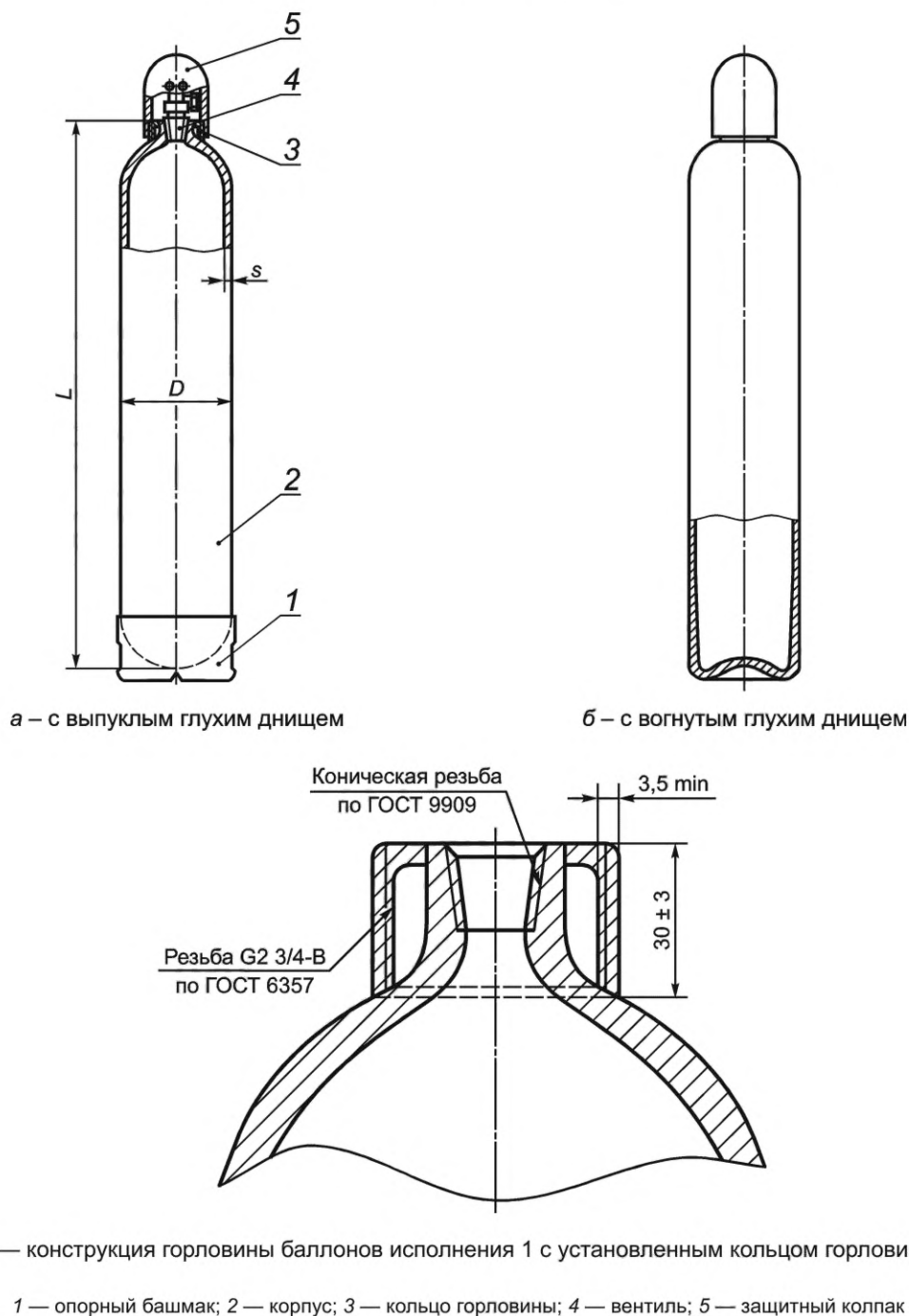
Рисунок 1 — Типовая конструкция баллонов
