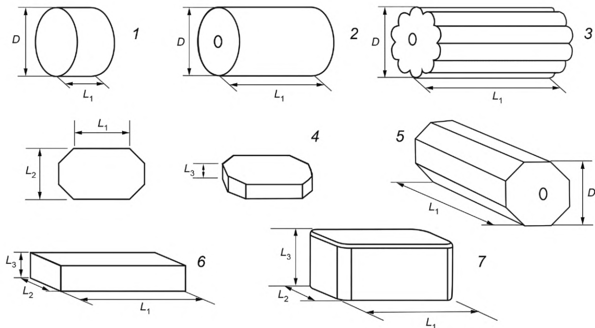
Рисунок 1 — Размеры брикетов
