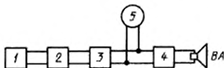
1 — генератор белого или розового шума ГШН; 2 — фильтр ФПНМ; 3 — усилитель мощности У2; 4 — эквивалентный фильтр, параметры которого приведены в ТУ; 5 — электронный вольтметр; ВА — контролируемый громкоговоритель
