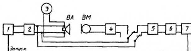
1 – генератор импульсов; 2 – усилитель мощности У1; 3 – универсальный осциллограф; 4 – микрофонный усилитель УМ; 5 – фильтр нижних частот ФНЧ; 6 – ана- лого-цифровой преобразователь АЦП; 7 – процессор
