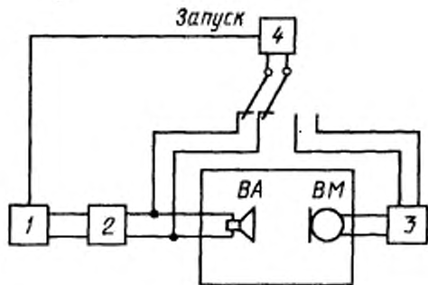
1 — генератор импульсов; 2 — усилитель мощности У1; 3 — микрофонный усилитель УМ; 4 — универсальный осциллограф; ВА — контролируемый громкоговоритель; ВМ — измерительный микрофон
