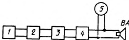
1 — генератор белого или розового шума ГШН; 2 — фильтр ФПШМ; 3 — фильтр ФЗД; 4 — усилитель мощности У2; 5 — электронный вольтметр; ВА — контролируемый громкоговоритель
