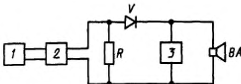
1 — импульсный генератор; 2 — усилитель мощности У1 или У2; 3 — универсальный осциллограф; V — полупроводниковый диод; R — резистор с сопротивлением 100 Ом ± 20 %; BA — контролируемая головка громкоговорителя
