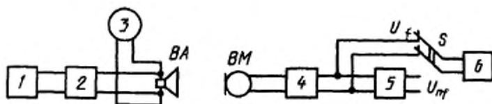
1 – генератор ГНИ; 2 – усилитель мощности У1; 3 – электронный вольтметр; 4 – микрофонный усилитель УМ; 5 – фильтр ФВЧ; 6 – универсальный осциллограф; ВМ – микрофон для измерения призвука и дребезжания; ВА – контролируемый громкоговоритель; S – переключатель
