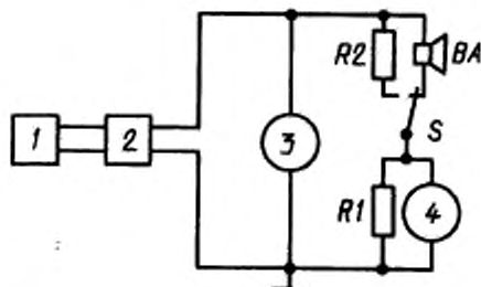
1 — генератор ГНИ; 2 — усилитель мощности У1; 3, 4 — электронные вольтметры; R1, R2 — резисторы; BA — контролируемый громкоговоритель; S — переключатель
