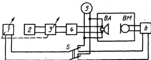
1 – регистрирующее устройство; 2 – генератор розового шума ГПН; 3 – переключаемый узкополосный фильтр; 4 – усилитель мощности У1; 5 – электронный вольтметр; 6 – микрофонный усилитель УМ; BA – контролируемый громкоговоритель; BM – измерительный микрофон
