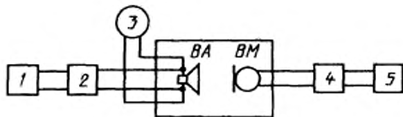
1 — генератор ГНИ; 2 — усилитель мощности У1; 3, 5 — электронный вольтметр; 4 — микрофонный усилитель УМ; BA — контролируемый громкоговоритель; BM — измерительный микрофон
