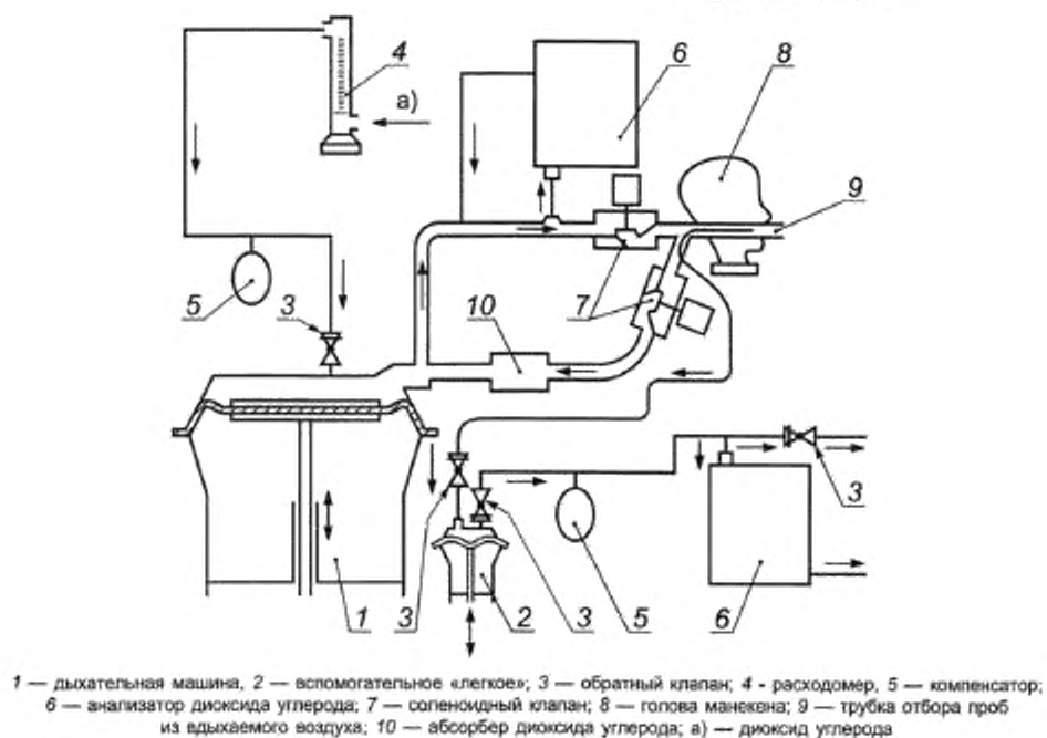
Рисунок 3 — Испытательная установка для определения содержания диоксида углерода
