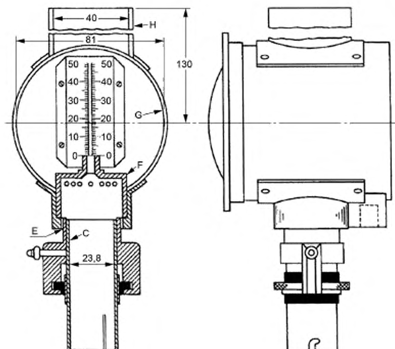
Примечание 1 — Размеры в миллиметрах.
