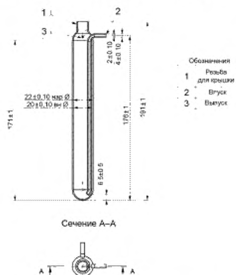
Рисунок А.3 — Испытательный сосуд
